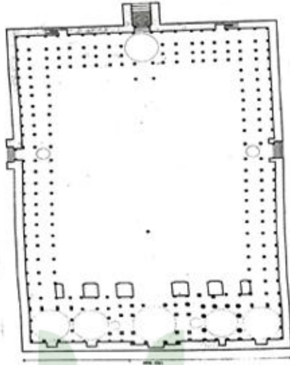
مسقط افقي يوضح الطراز الاول لمسجد قبة الاسلام
